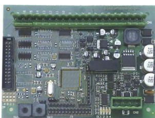
STG/OUT16-S
